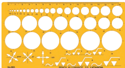
012-0020 No.865 円定規 .....1,300 円(税込 1,430 円) 包装入数 1/30 ●180×96mm ●厚さ0.8mm ●直径0.8~28mm ●33穴 ●ブチレート製
