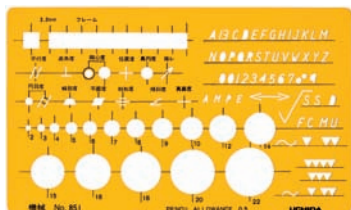
1-843-0851 No.851 機械定規 .....1,280 円(税込 1,408 円) 包装入数 1/40 ●159×95mm ●厚さ0.6mm ●文字高4mm ●ブチレート製
