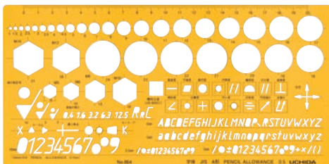
012-0019 No.864 機械記号定規 .....1,640 円(税込 1,804 円) 包装入数 1/30 ●233×114mm ●厚さ0.8mm ●直径1~24mm ●28穴 ●文字高 英字5.0mm 数字3.5mm 5mm 10mm ●文字内容: A形斜体 ●ブチレート製
