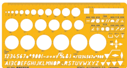
012-0023 No.868 機械科用定規 .....1,300 円(税込 1,430 円) 包装入数 1/30 ●180×96mm ●厚さ0.8mm ●直径1~24mm ●24穴 ●文字高 英字5mm 数字3.5mm 5mm ●文字内容: A形斜体 ●ブチレート製
