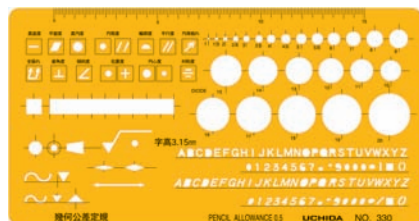
1-843-1808 No.330M 幾何公差定規 インキエッジ付き ..... 1,640 円(税込 1,804 円) ●200×105mm ●厚さ0.8mm ●文字高3.15mm ●ブチレート製 ●文字内容：B形直立体 斜体 JISZ813製図用 包装入数 1/30
