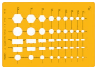
1-843-0301 No.301 ボルトナット定規 ..... 1,280 円(税込 1,408 円) ●193×135mm ●厚さ0.8mm ●穴径JIS M3～M12 ●5種 45穴 ●ブチレート製 包装入数 1/30
